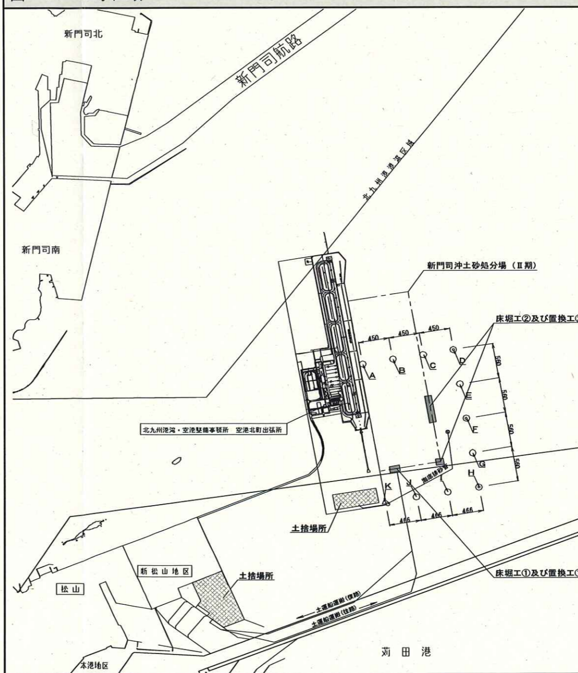
図-1. 工事区域
