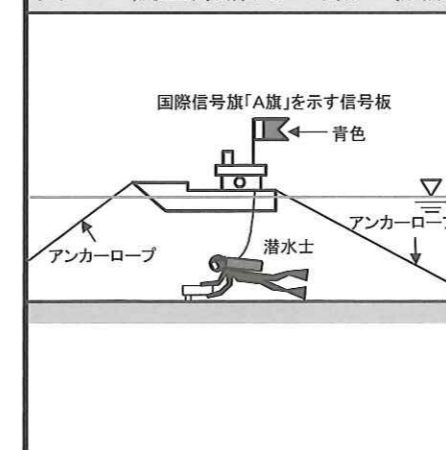
図-2 調査船(潜水士船)の標識
