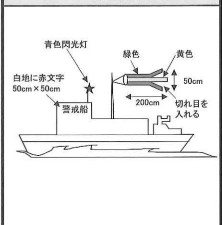
図-4 警戒船の標識
