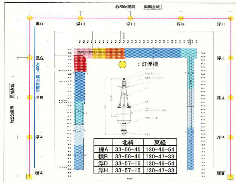
図-2 護岸築造工事平面図
