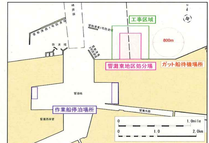
図-6 作業船停泊場所図
