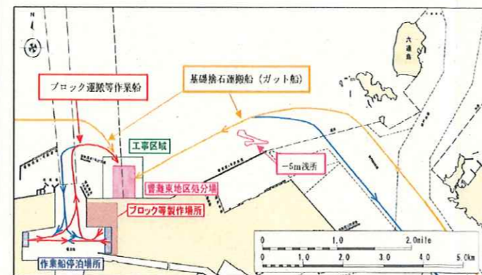
図-3 石材運搬経路図
