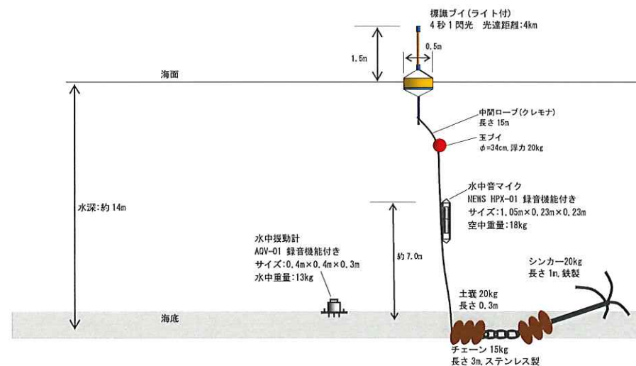
図-2 水中騒音海底振動測定状況
