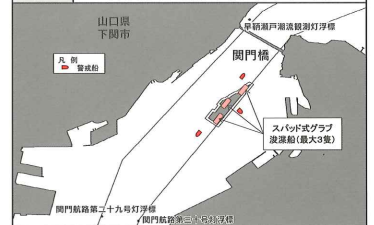
図-5 浚渫船・警戒船配置図【浚渫時の例】
