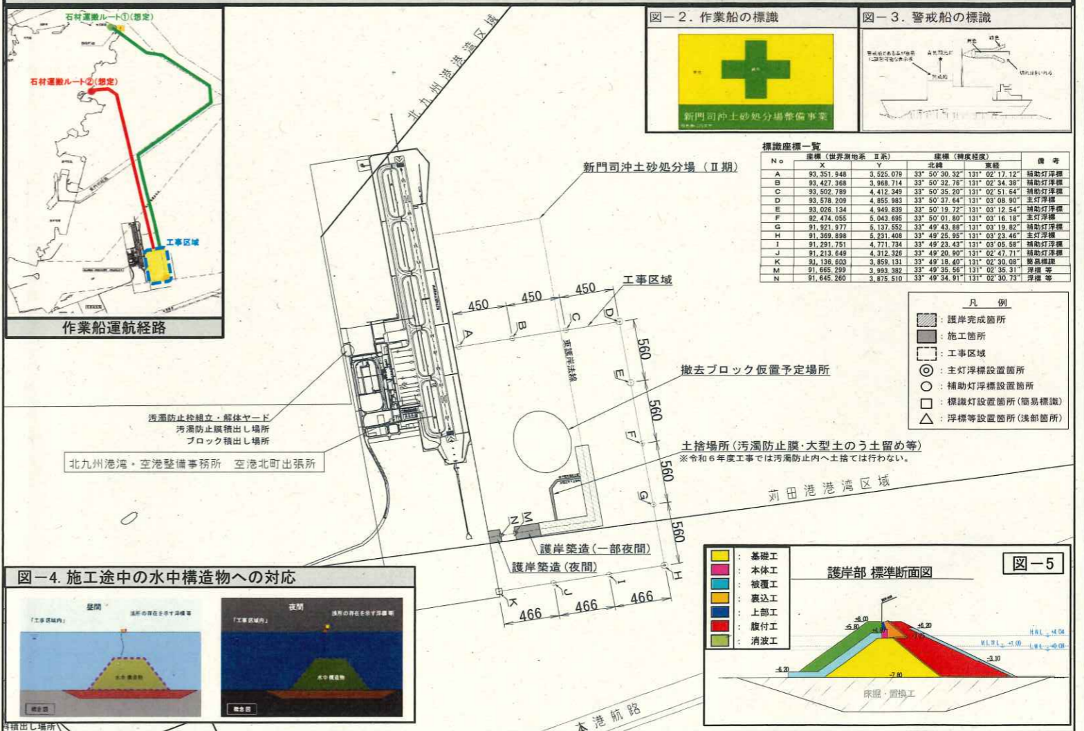
図-1. 工事区域
