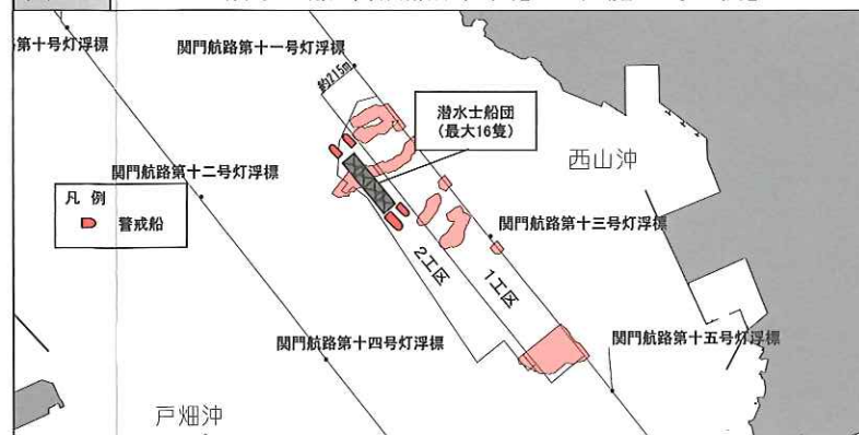
図-3 潜水士船・警戒船配置図【2工区施工時の例】
