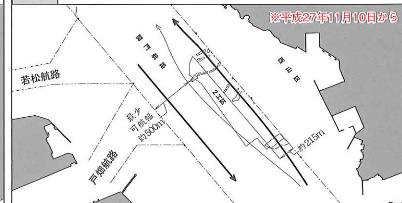
図-5 2工区施工時の通航方法
